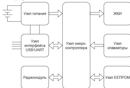
Рисунок 1 Структурная схема устройства
