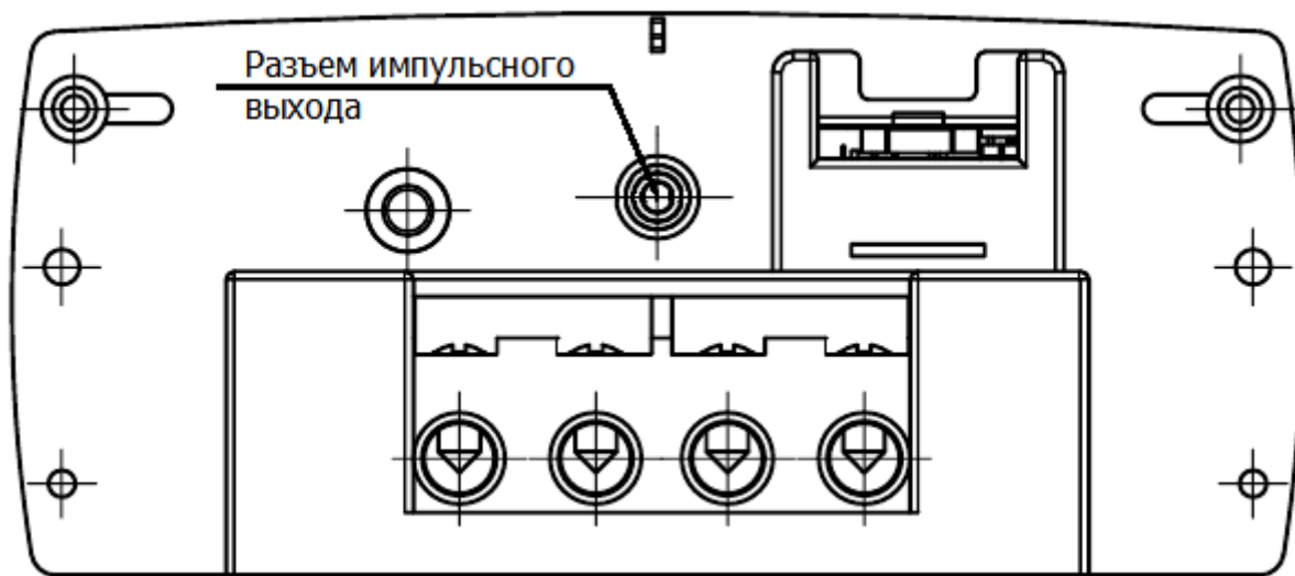
Рисунок 3. Обозначение функциональных контактов счетчика
