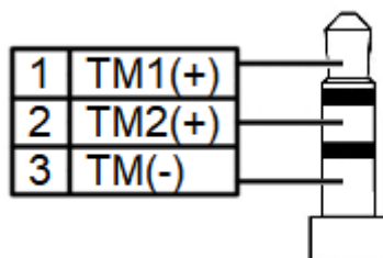
Рисунок 4. Схема подключения импульсного выхода
