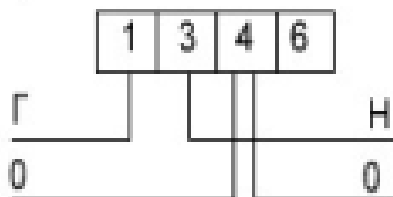
Рисунок 2.1. Схема подключения счетчика
