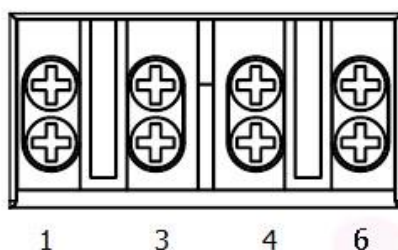
Рисунок 4. Обозначение контактов зажимов счетчика
