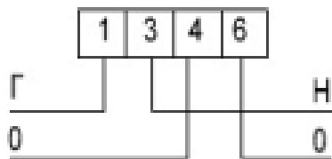
Рисунок 2.1. Схема подключения счетчика
