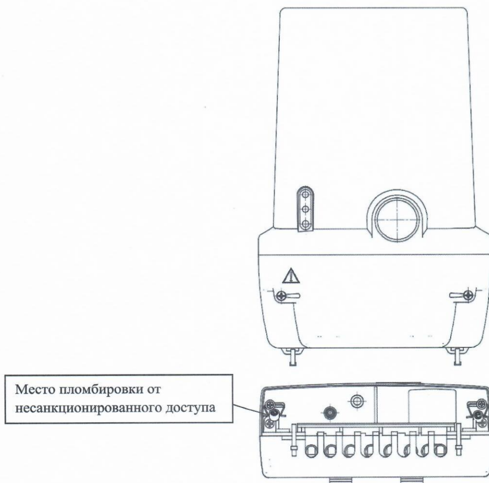
Рисунок 3.6 - Схема (рисунок) с указанием мест пломбировки от несанкционированного доступа на счетчик СЕ318ВУ СЗ
