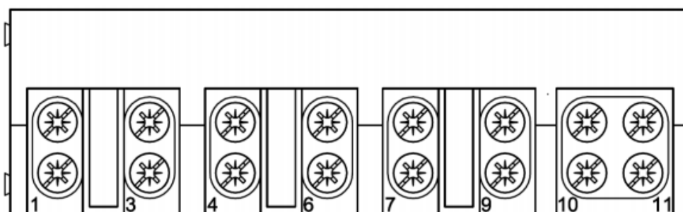
Рисунок 13. Обозначение контактов зажимов счетчика СЕ318 исполнения с максимальным током 100 А
