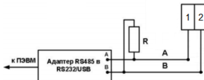
Рисунок 17. Схема подключения интерфейса RS-485 счетчика CE318 R32
