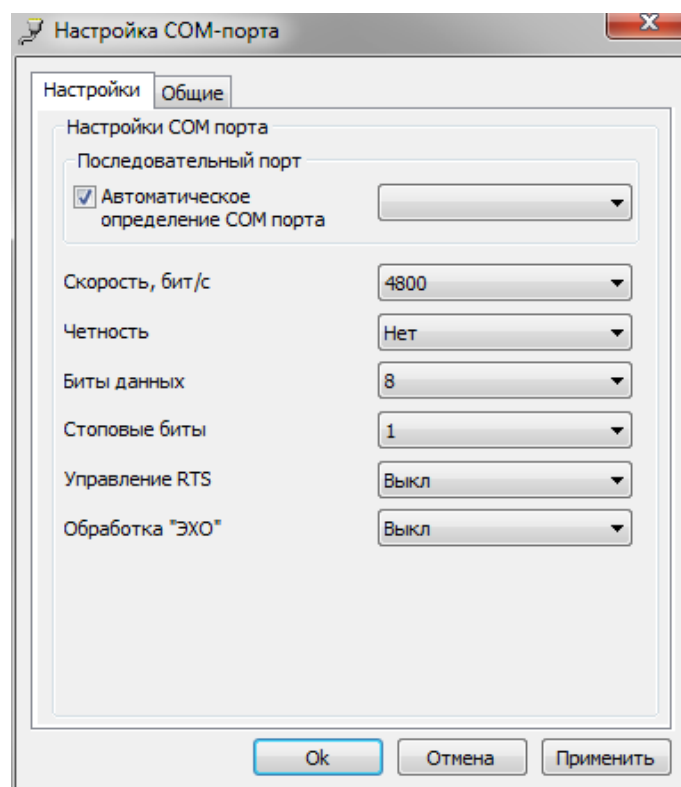
Рисунок 29. Настройки канала связи «RS232»
