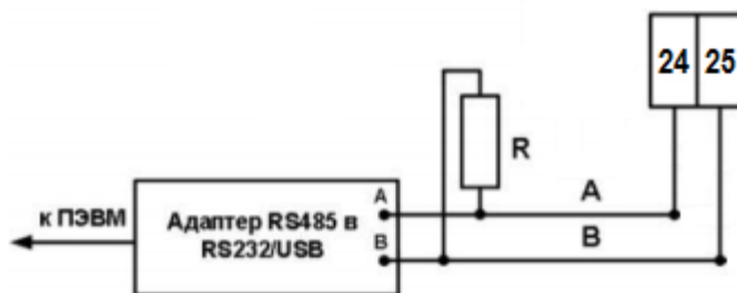
Рисунок 20. Схема подключения интерфейса RS-485 счетчика CE318 S35
