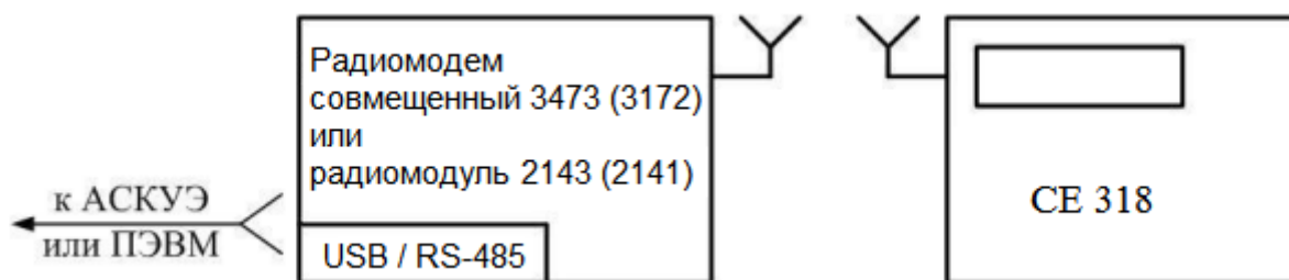
Рисунок 21. Схема подключения счетчика через радио-интерфейс
