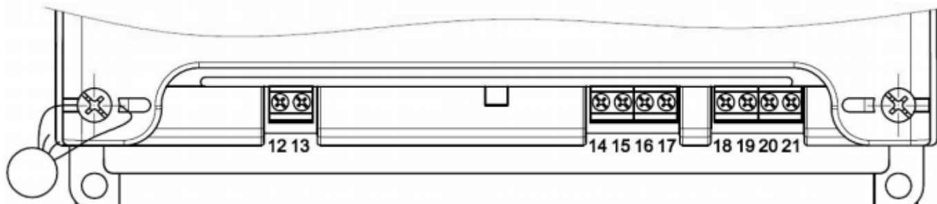
Рисунок 7. Обозначение функциональных контактов счетчика CE318 R32
