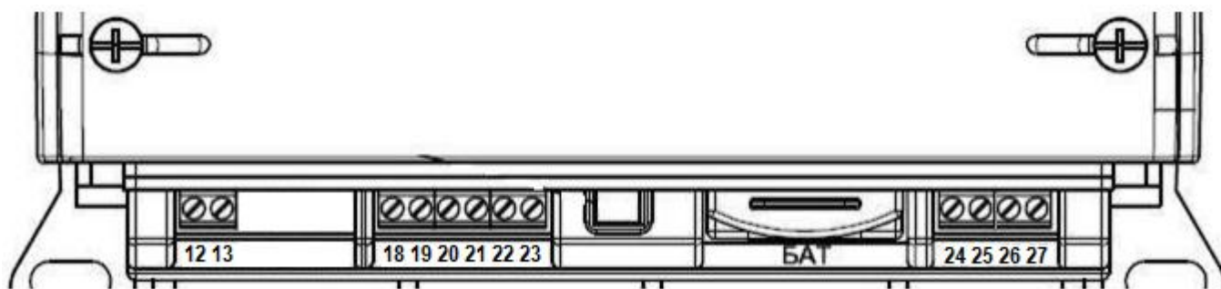
Рисунок 9. Обозначение функциональных контактов счетчика СЕ318 S35 трансформаторного по току включения
