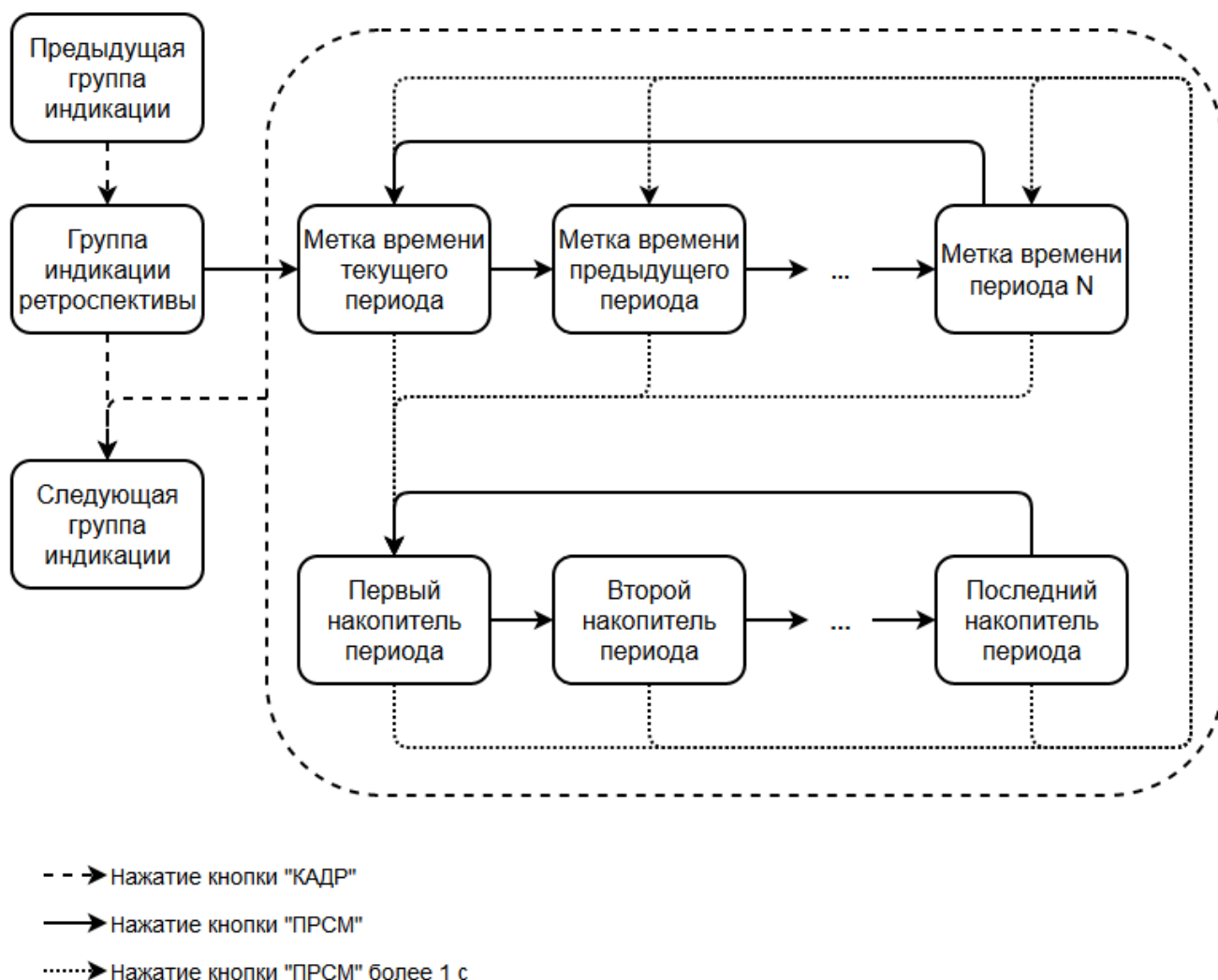
Рисунок 52 Блок-схема просмотра ретроспективы для счетчиков (идентификатор устройства 148)
