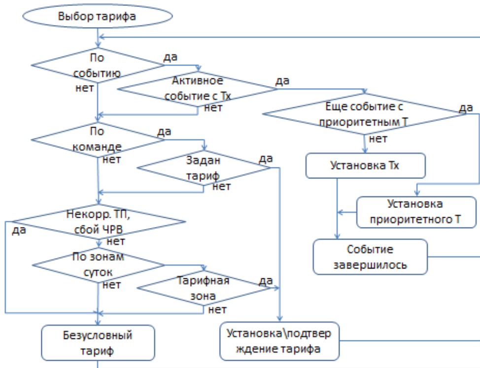
Рисунок 54. Алгоритм выбора действующего тарифа
