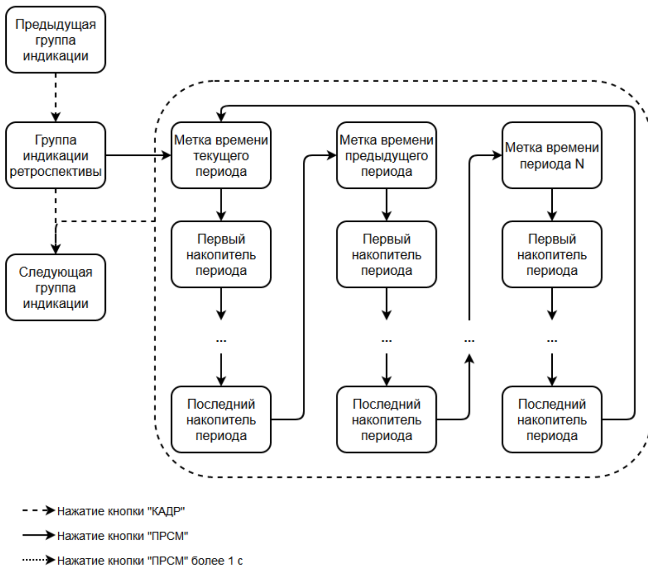
Рисунок 51 Блок-схема просмотра ретроспективы для счетчиков (идентификатор устройства 94)
