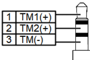
Рисунок 15. Схема подключения импульсного выхода
