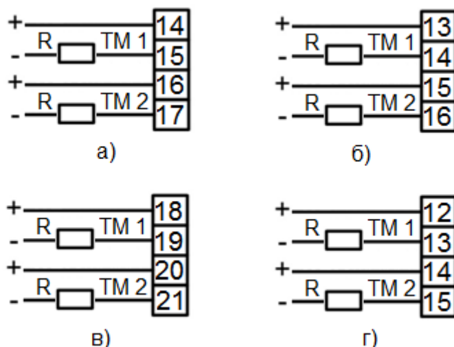
Рисунок 14. Схема подключения импульсного выхода
