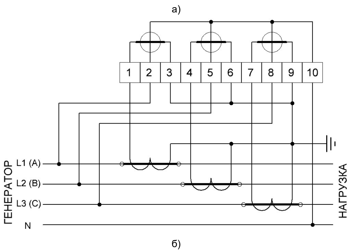
Рисунок 4. Схемы подключения счетчика СЕ318 полукосвенного включения. Подключение через три трансформатора тока, трехфазная четырехпроводная сеть
