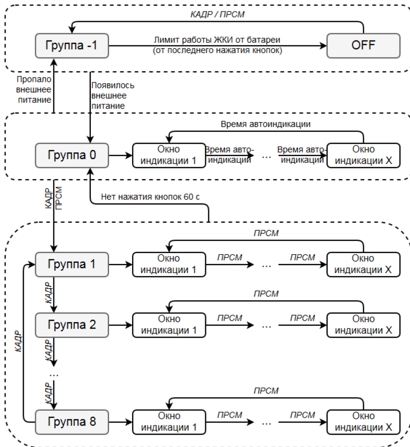
Рисунок 38. Алгоритм переключения групп индикации
