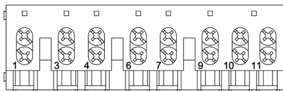
Рисунок 12. Обозначение контактов зажимов счетчика СЕ318 исполнения с максимальным током 60 или 80 А
