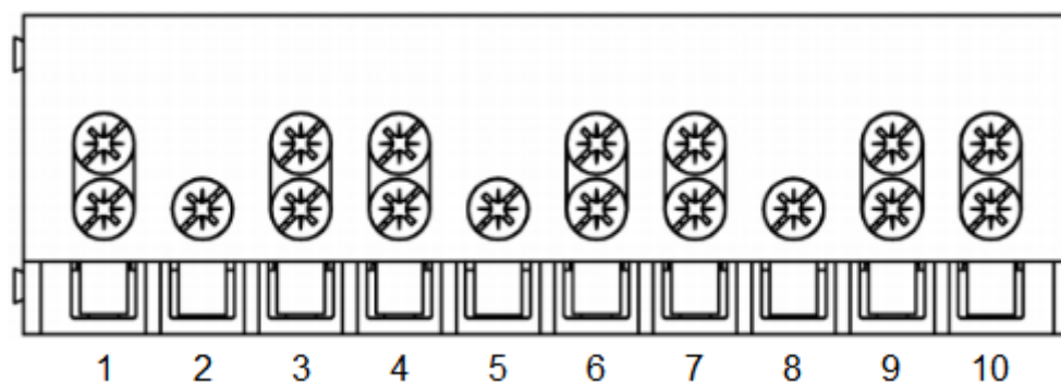
Рисунок 11. Обозначение контактов зажимов счетчика СЕ318 трансформаторного по току включения
