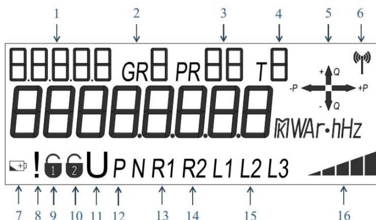
Рисунок 39. Символы и знаки, отображаемые на ЖКИ
