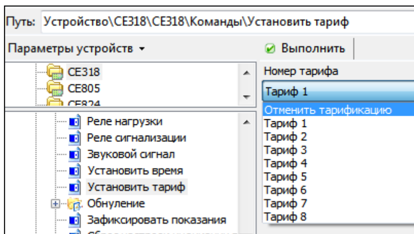
Рисунок 56. Управление тарификацией в режиме внешней тарификации
