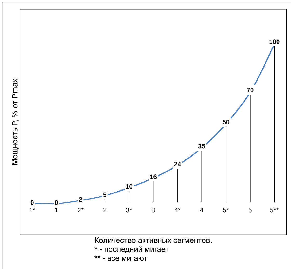
Рисунок 40. Зависимость индикатора активной мощности от фактического уровня активной мощности
