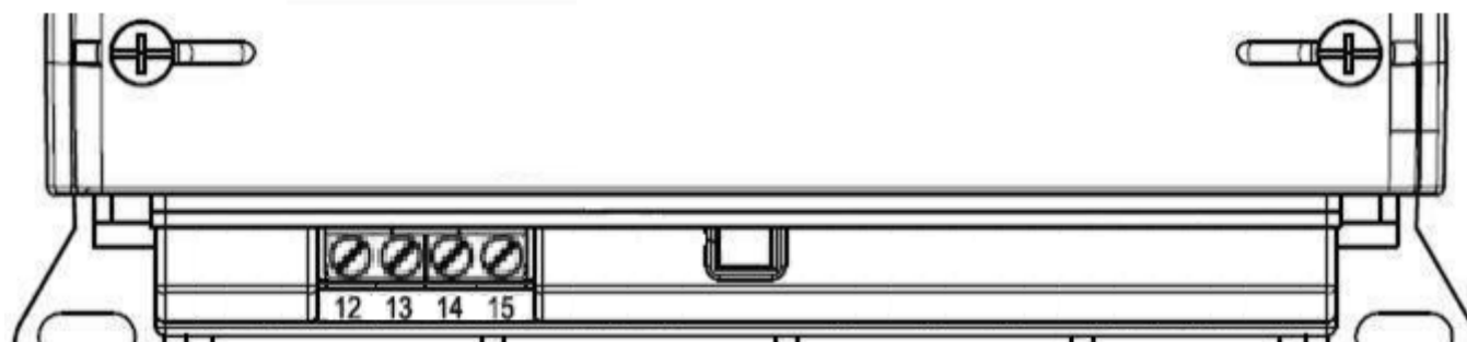
Рисунок 10. Обозначение функциональных контактов счетчика СЕ318 S35 непосредственного включения
