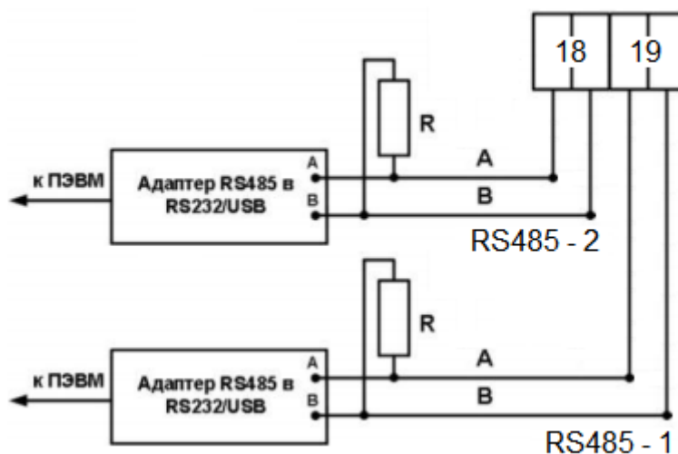
Рисунок 19 Схема подключения интерфейсов RS-485 счетчика CE318 S31, исполнения с двумя интерфейсами RS-485
